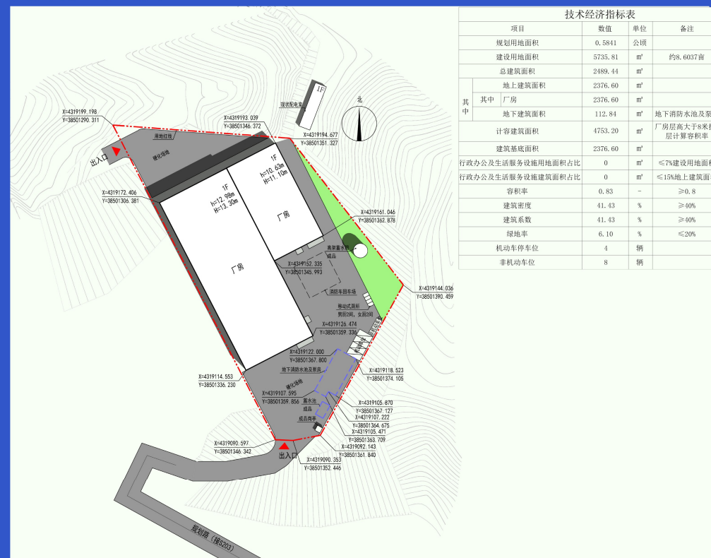
变更后总平面图
