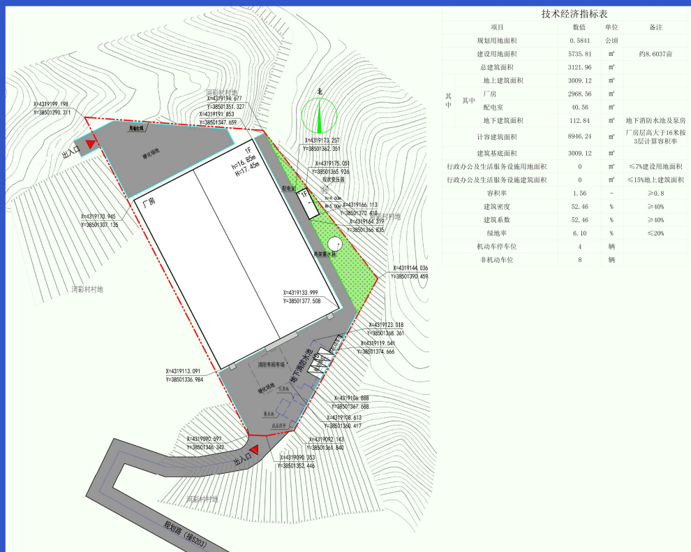
变更前总平面图
